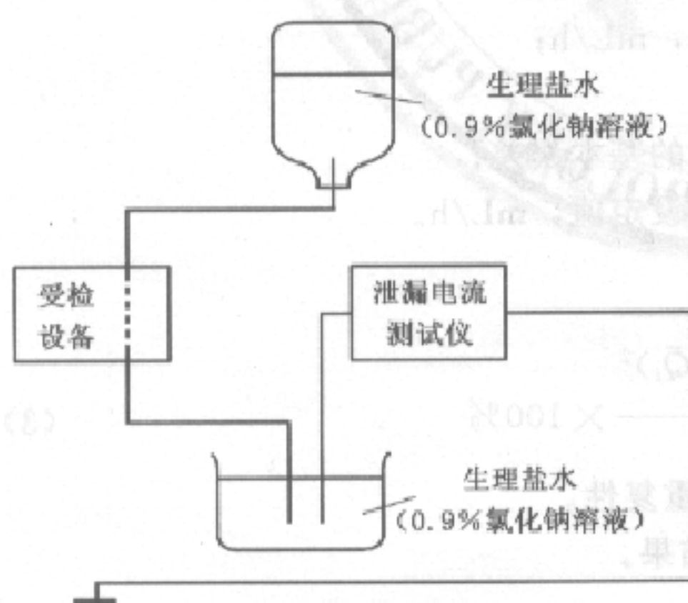
图 1 患者漏电流—外部电源供电
