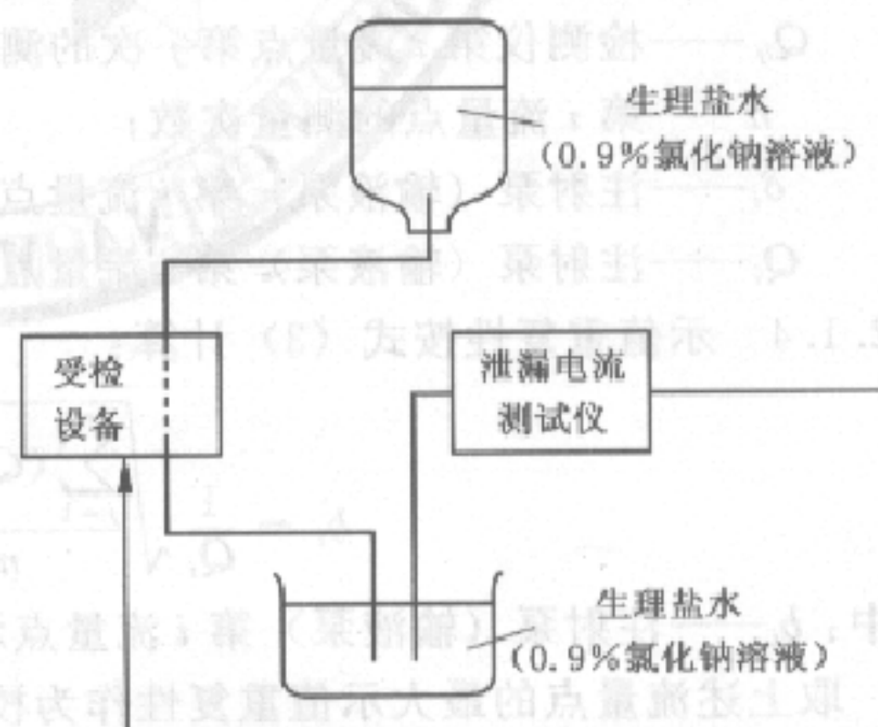
图 2 患者漏电流—内部电源供电
